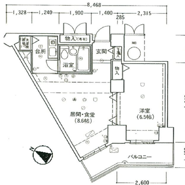
図3~15階平面図
